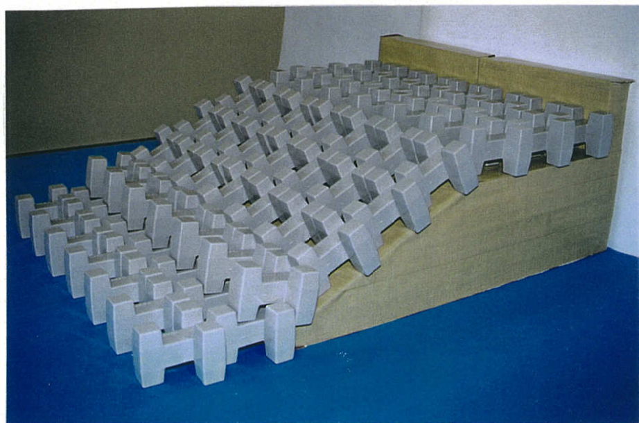
斜面被服工 (正積)
